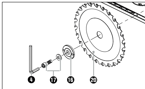
Slika A: Zamena lista testere
