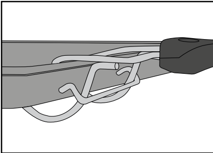
2. ábra: A fogó 10 beakasztása a sütőlemez 9
