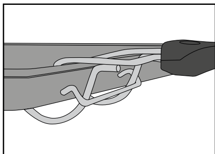
Rys. 2: Zaczepianie szczypecie 10 za pieczenia 9
