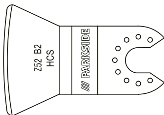
Schaafmes Z52 B2 ①
