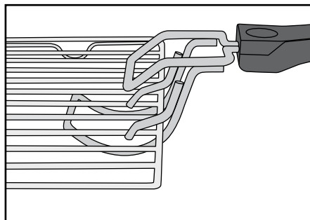
Fig. 4 : Accrochage de la pince ⑩ avec la grille ⑬
