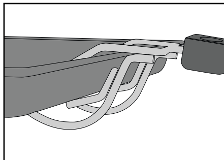
Fig. 5 : Accrochage de la pince ⑩ avec le plateau ⑪.
