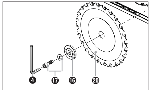
Εικ. Α: Αλλαγή λεπίδας πριονιού
