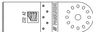
pânză interschimbabilă HCS 95 x 32 mm
