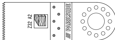
Uranjajući list pile (32 mm) Z32 A2 [6]
