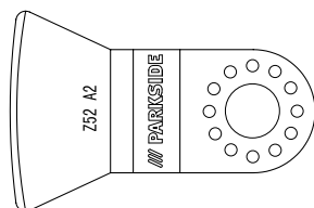
Cuchilla de raspado Z52 A2 [9]
