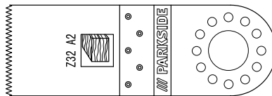
Lâmina de serra de imersão (32 mm) Z32 A2 6
