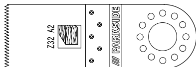
Brzeszczot węgłny (32 mm) Z32 A2 [6]
