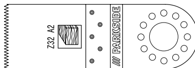
Invalzaagblad (32 mm) Z32 A2 6
