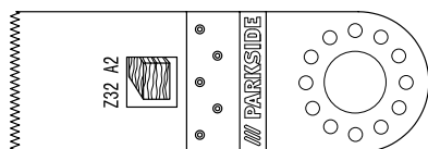
Upotussahanterä (32 mm) Z32 A2 [6]
