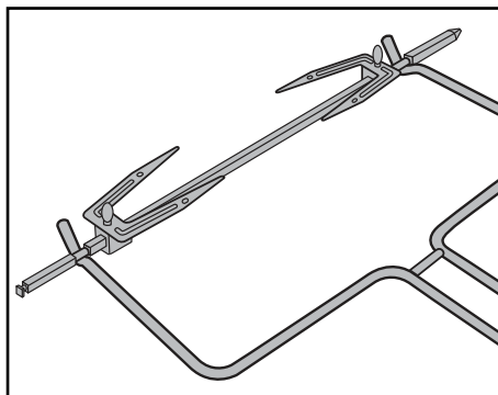
Fig. 3 : Accrochage de la pince 12 avec le tournebroche 16
