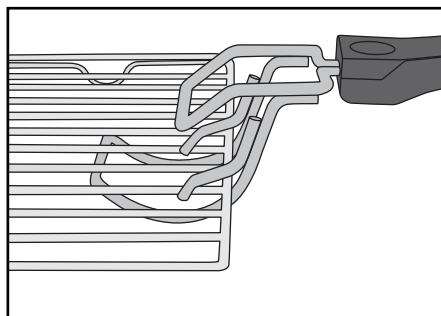
Abb. 4: Einhängen der Zange ⑩ beim Gitterrost ⑬
