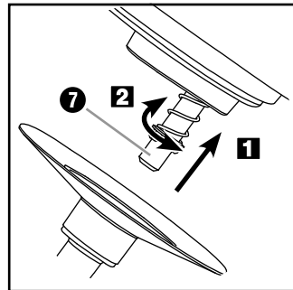
Obr. 2: Montáž nadstavcov
