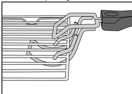
Fig. 4: Aggancio della pinza 10 alla griglia 13
