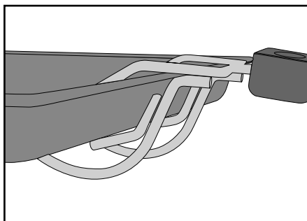
Fig. 5: Aggancio della pinza 10 alla teglia da forno 11
