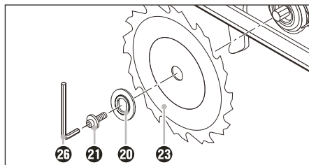
Фиг. А: Смяна на циркулярен диск
