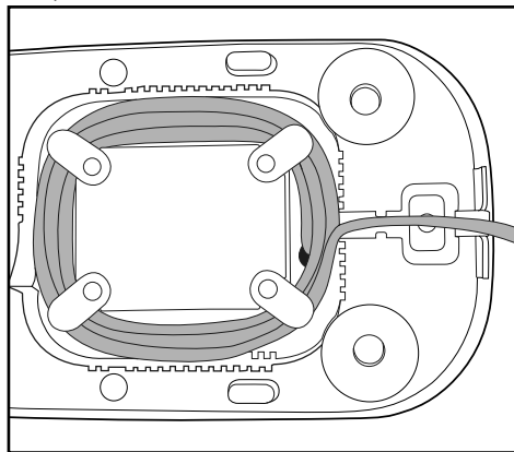
Afb. 3: Kabelspoel
