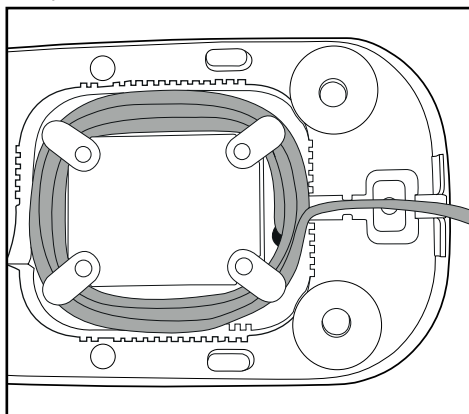
3. ábra: Kábelszévelő
