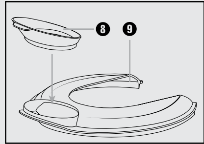
Фиг. 2: Монтаж на помощното приспособление за пълнене
