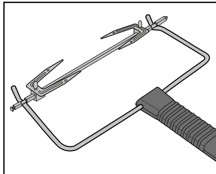
Obr. 3: Zakvačenie klieští 12 pri otočnom ražni 16
