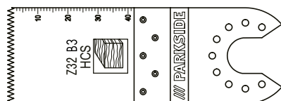
Потопящ се режещ нож HCS 32 mm
