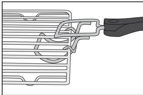
Rys. 1: Zaczepianie szczypiec 10 za ruszt 8
