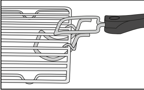
Fig. 1 : Accrochage de la pince 10 avec la grille 8
