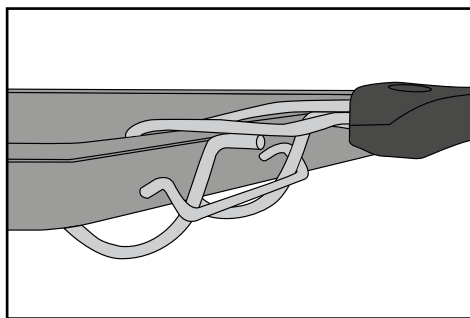
Obr. 2: Zaháknutie klieští 10 pri plechu na pečenie 9
