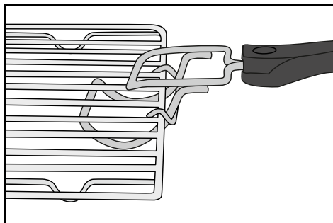
Obr. 1: Zaháknutie klieští 10 pri mriežkovom rošte 8
