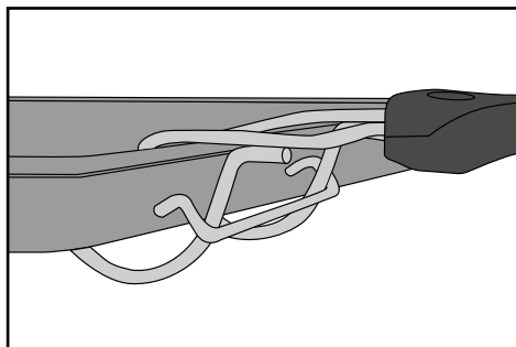
Fig. 2: Aggancio della pinza 10 alla teglia da forno 9
