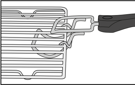
Fig. 1 : Accrochage de la pince 10 avec la grille 8
